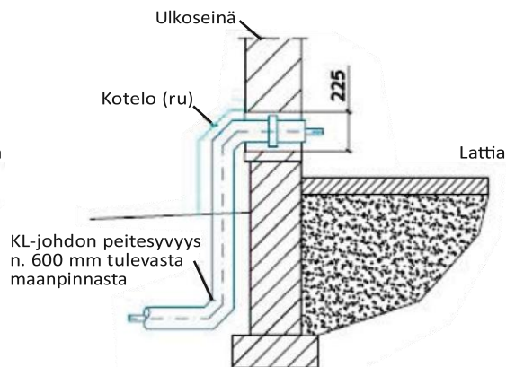
PERUSMUURIN ULKOPUOLINEN ASENNUS:
