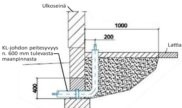
PERUSMUURIN AUKKO:
