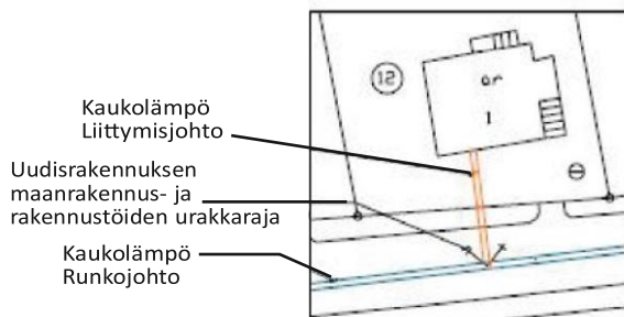
KAUKOLÄMPÖLIITTYMÄ:
