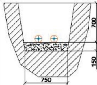
LIITTYMISJOHDON KAIVANTO:
